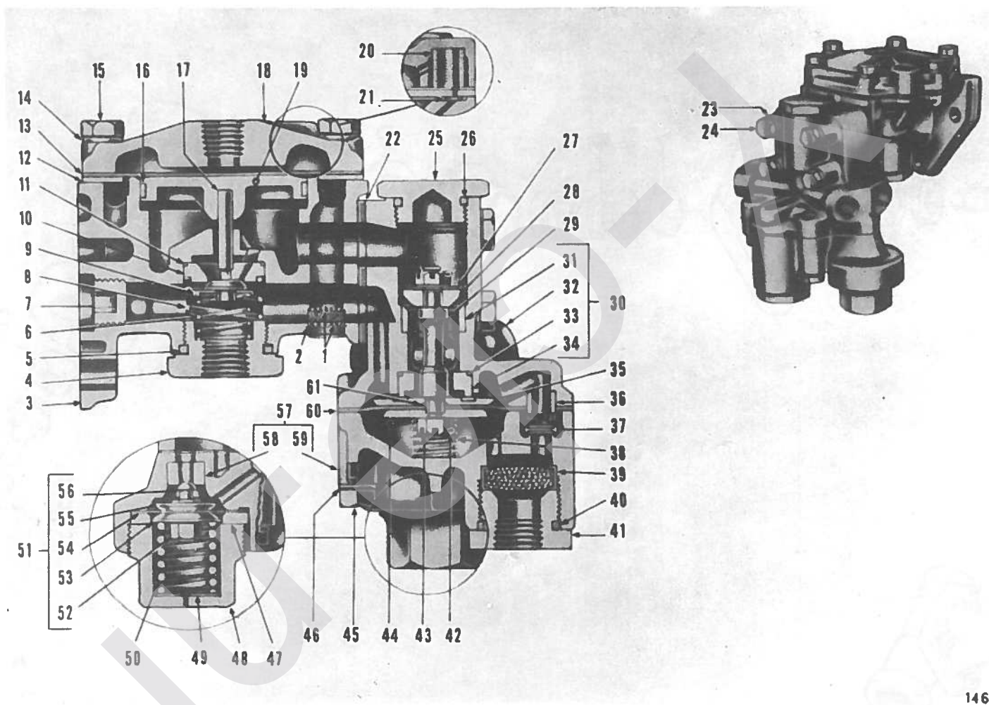
2 DL - AFB 1206 - REACTIE-VEILIGHEIDSVENSTIEL 3/5 DL
