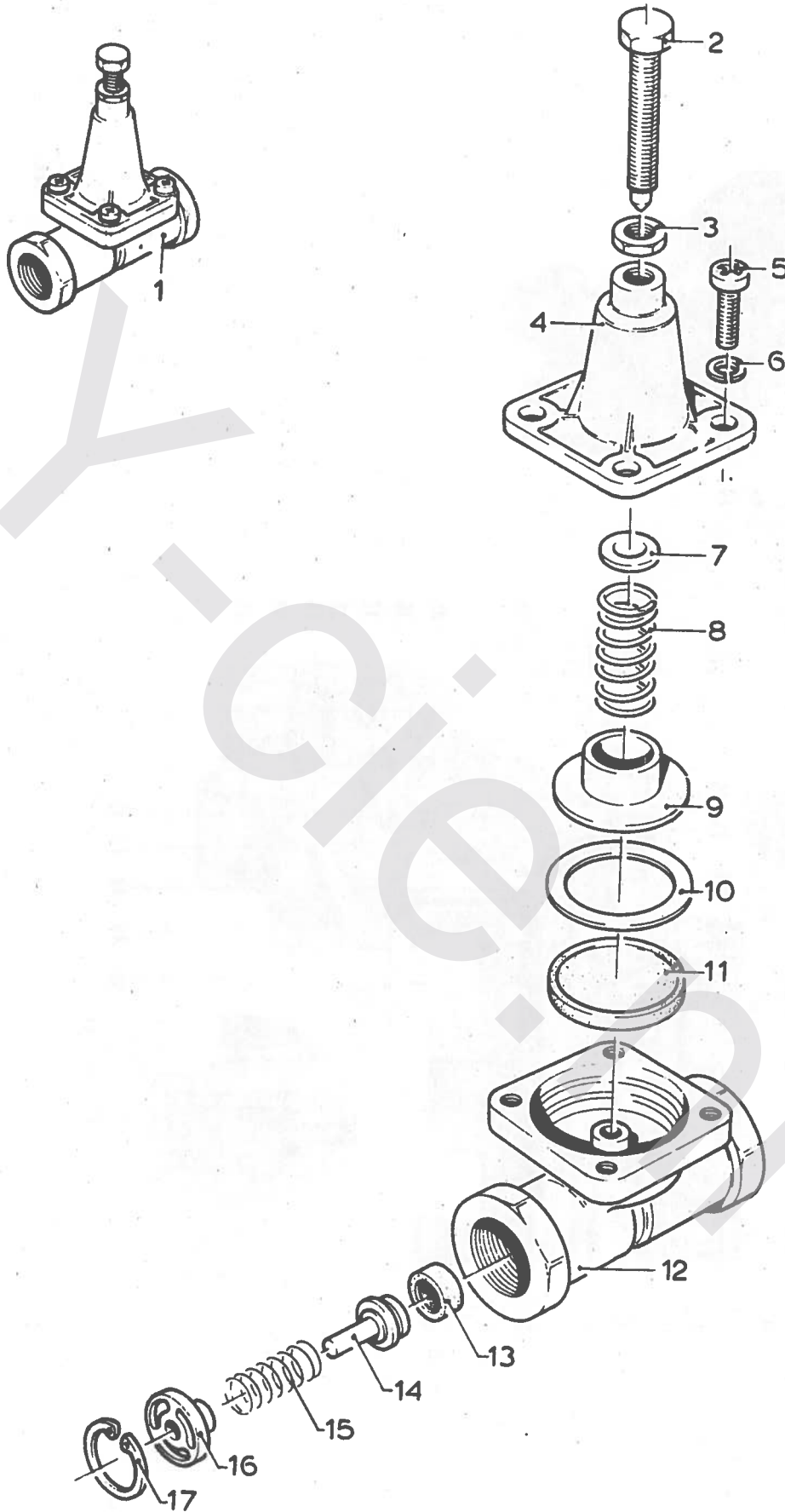
2 DL 3/5 DL - AFB 1205 - OVERSTROOMVENTIEL
